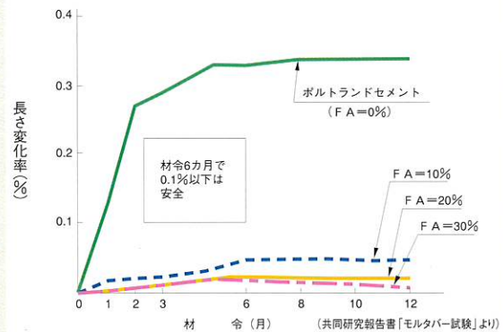
フライアッシュ使用により、モルタルの膨張が1/20となり、アルカリシリカ反応がほぼ完全に抑制された例
